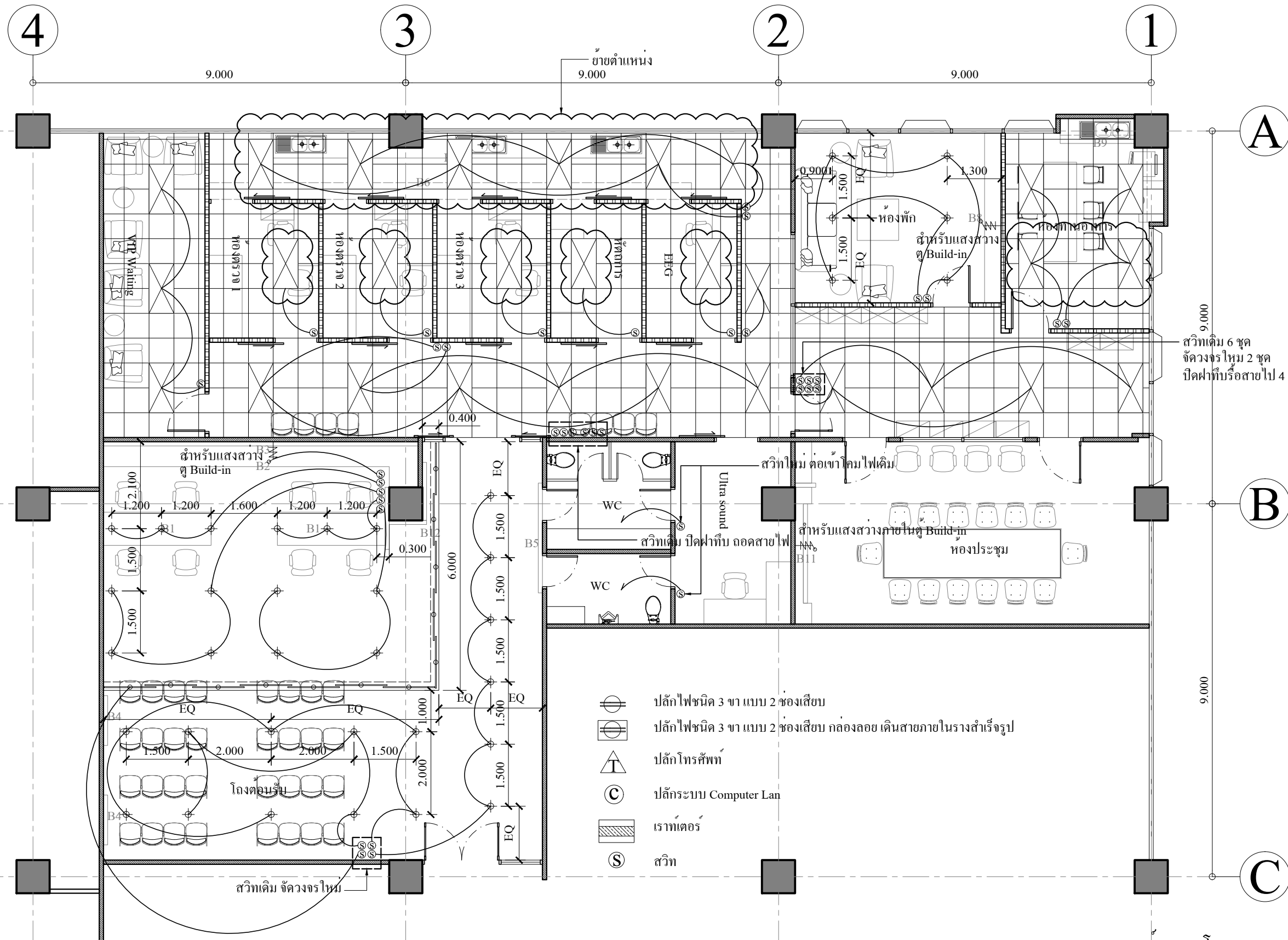
ศูนย์สมอง โรงพยาบาลสมเด็จพระปิ่นเกล้า ผังฟ้าและระบบแสงสว่างใหม่ Scale 1:100
